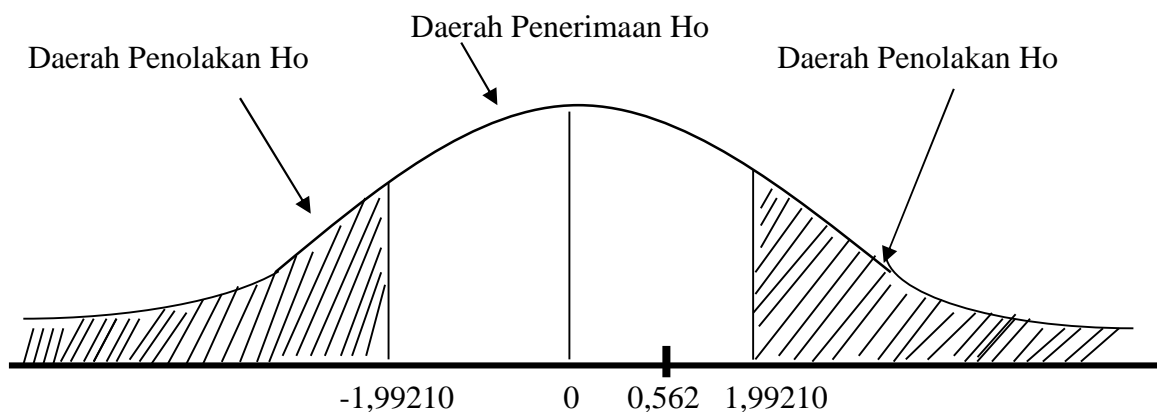
Gambar 6 :Kurva normal uji t
