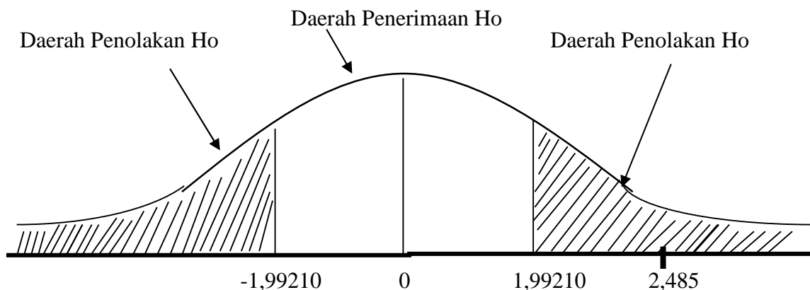
Gambar 7 : Kurva normal uji t
